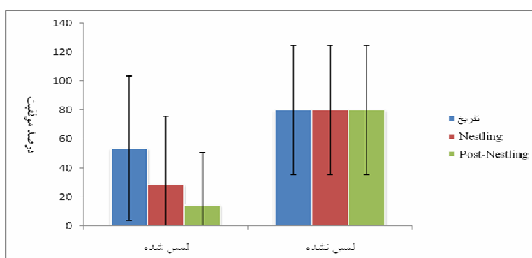
نمودار ۳ - مقایسه میانگین درصد موفقیت در مراحل مختلف جوجه‌آوری یاکریم (Mean±SD).
