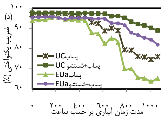
شکل ۵- روند تغییرات ضرایب یکنواختی پخش مطلق (EU a ) و یکنواختی کریستیان سن (UC) چهار نوع قطره‌چکان مورد آزمایش در شرایط استفاده از
