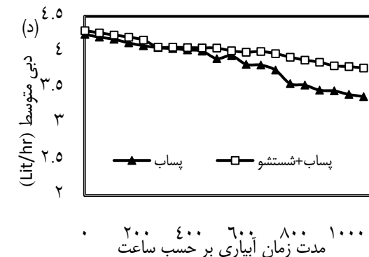
شکل ۱- روند تغییرات آبدهی چهار نوع قطره‌چکان در شرایط استفاده از پساب تصفیه‌شده و پساب همراه
