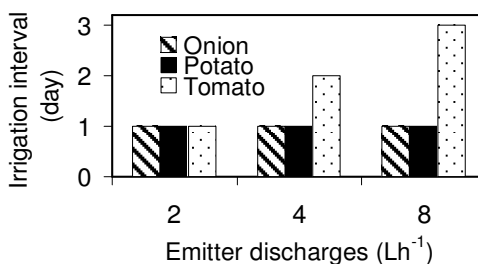
شکل ۷- دور آبیاری با کاربرد دبی‌های ۲ تا ۸ لیتر (لیتر بر ساعت) برای آبیاری گیاهان مختلف
