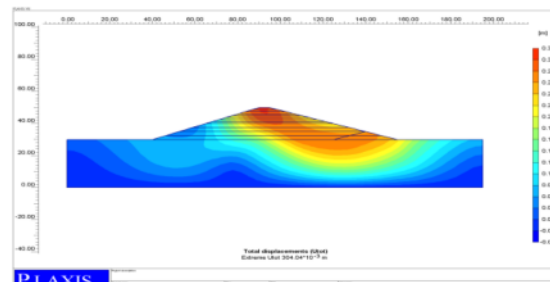
شکل ۱۶. تغییر شکل کلی در آنالیز مربوط به آبگیری سد خاکی همگن به ارتفاع ۱۹ متر پس از تحکیم (حداکثر ۳۰ سانتی متر)
