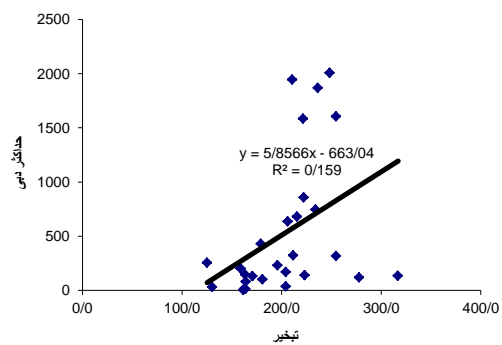
شکل ۷. رابطه و همبستگی مقادیر دما و تبخیر با ارتفاع و بارش متوسط سالانه در ۲۸ ایستگاه
