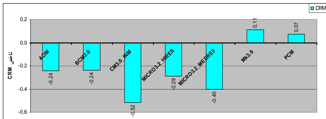
شکل ۱۸- مقایسه کمی بین مقادیر شاخص CRM در شبیه‌های GCM برای داده‌های دمای بیشینه.
