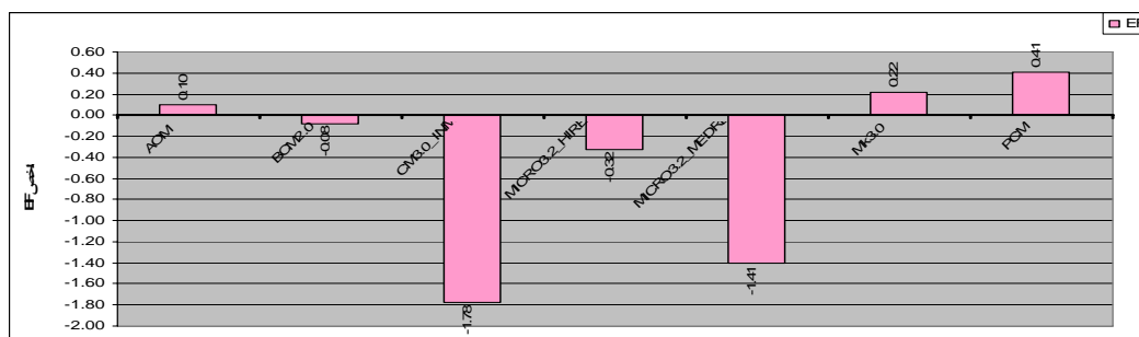
شکل ۱۷- مقایسه کمی بین مقادیر شاخص EF در شبیه‌های GCM برای داده‌های دمای بیشینه.
