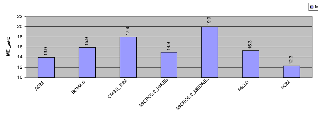
شکل ۱۴- مقایسه‌ی کمی بین مقادیر شاخص ME در شبیه‌های GCM برای داده‌های دمای بیشینه.
