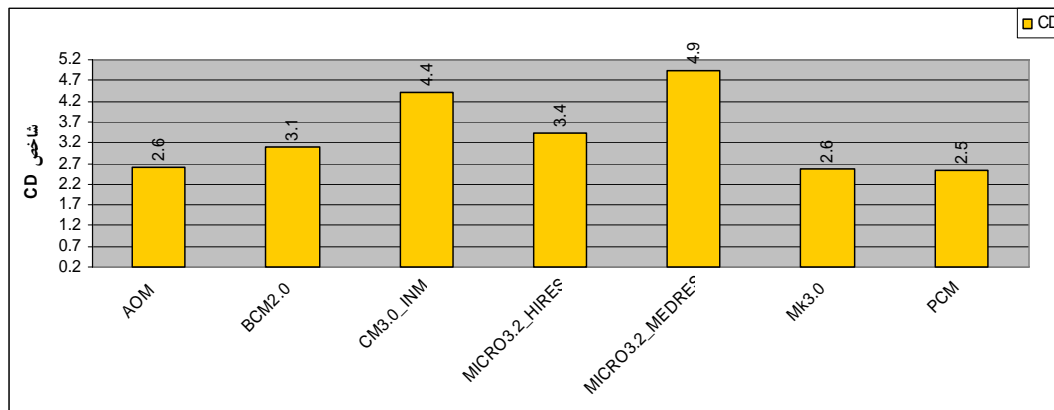
شکل ۱۶- مقایسه کمی بین مقادیر شاخص CD در شبیه‌های GCM برای داده‌های دمای بیشینه.
