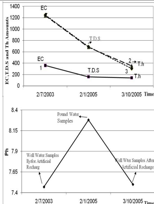
شکل شماره ۶- مقایسه مقادیر اسیدیته نمونه آب چاه های نیروگاه قبل (۱۳۸۲) و بعد از تغذیه (۱۳۸۴) و آب استخرهای تغذیه (۱۳۸۴) (چپ) و مقایسه هدایت الکتریکی، باقیمانده خشک و سختی کل نمونه های آب چاه های نیروگاه قبل از تغذیه (۳) و بعد از تغذیه (۲) و آب استخرهای تغذیه (۱) (راست).
