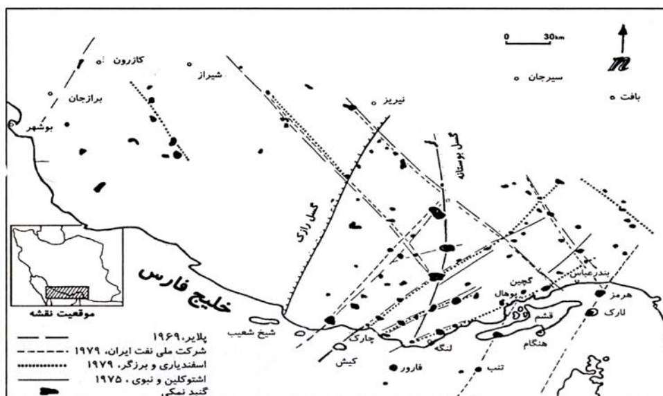
نقشه ۱: آرایش متفاوت گنبدهای نمکی منطقه بندرعباس - کازرون (نوی ای سبزه ای، ۱۳۶۹)
