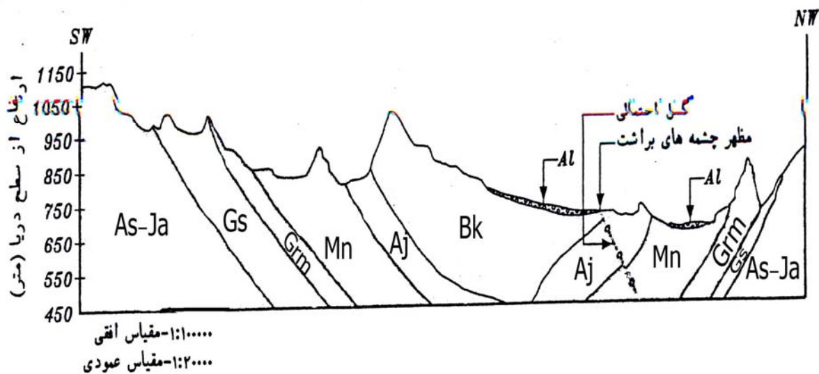
نقشه ۶ مقطع زمین شناسی محل مظهر چشمه های براشت
