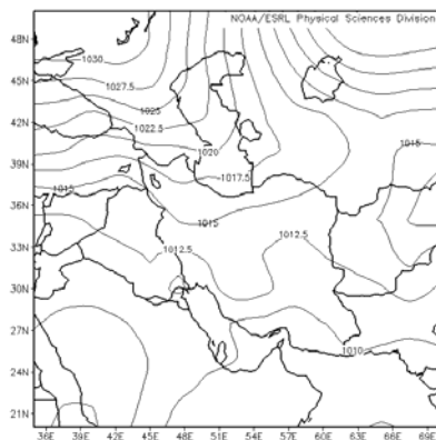
شکل ۷. سطح زمین (۱۶ اکتبر ۱۹۹۵)
