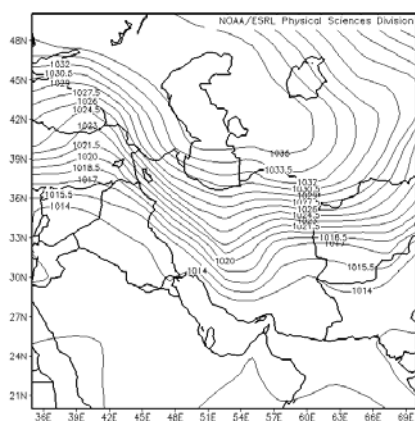
شکل ۹. سطح زمین (۱۷ اکتبر ۱۹۹۵)
