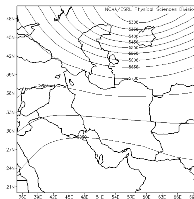
شکل ۸. سطح ۵۰۰ هکتو پاسکال (۱۶ اکتبر ۱۹۹۵)
