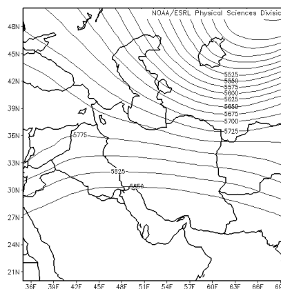
شکل ۱۰. سطح ۵۰۰ هکتوپاسکال (۱۷ اکتبر ۱۹۹۵)
