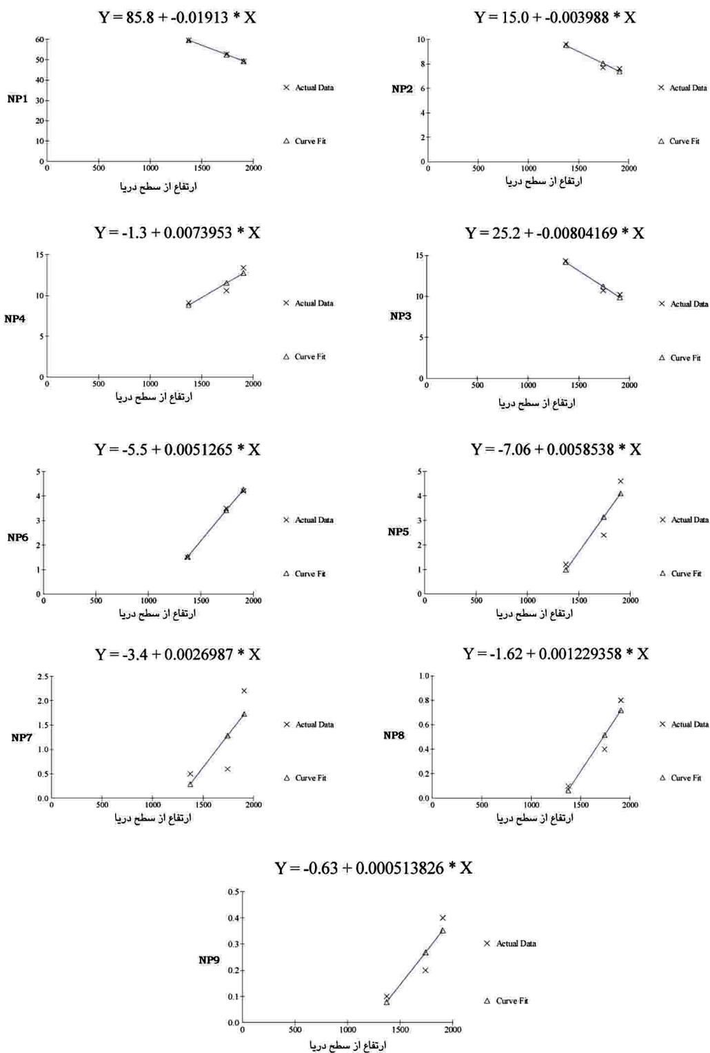
شکل ۳- روابط بین هر یک از احتمالات با ایستگاه‌های مختلف در مسیر سندیج- همدان
