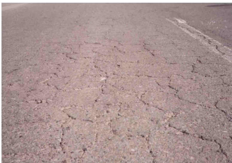
شکل ۲- تخریب روسازی آسفالت بر اثر یخبندان و تورم (محمودی، ۱۳۸۳)
