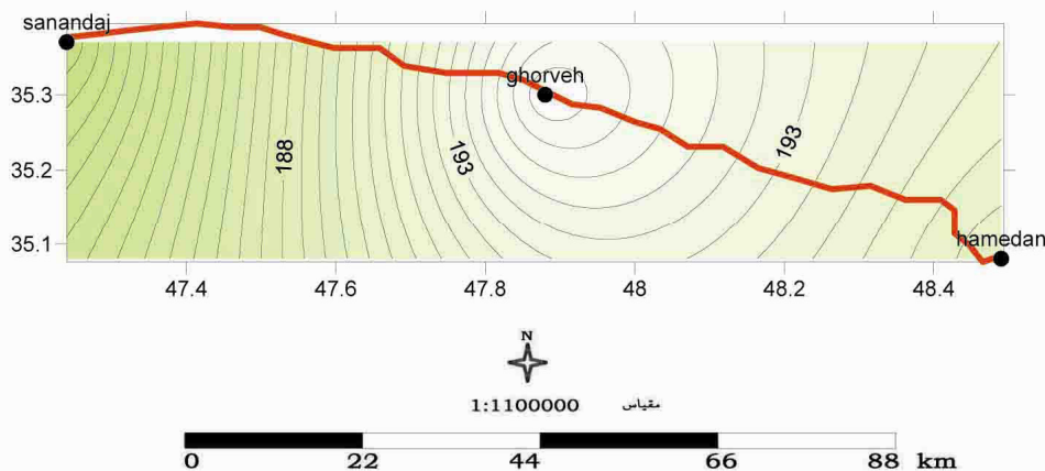
شکل ۱۴ - نقشه‌ی توزیع مکانی خاتمه یخبندان در مسیر سنندج - همدان
