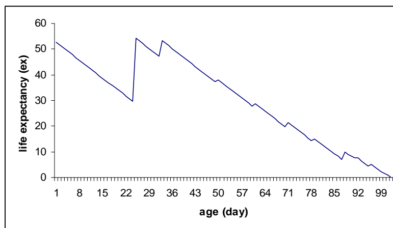
شکل ۲. منحنی امید زندگی ( e_x ) مگس میوه زیتون طی سنین مختلف
