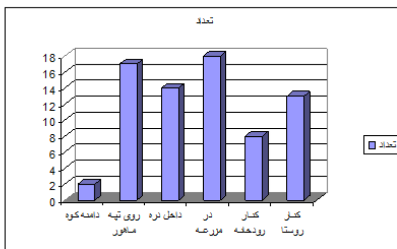
نمودار ۲: موقعیت محلی-زیست محیطی استقرارهای منطقه میربگ
