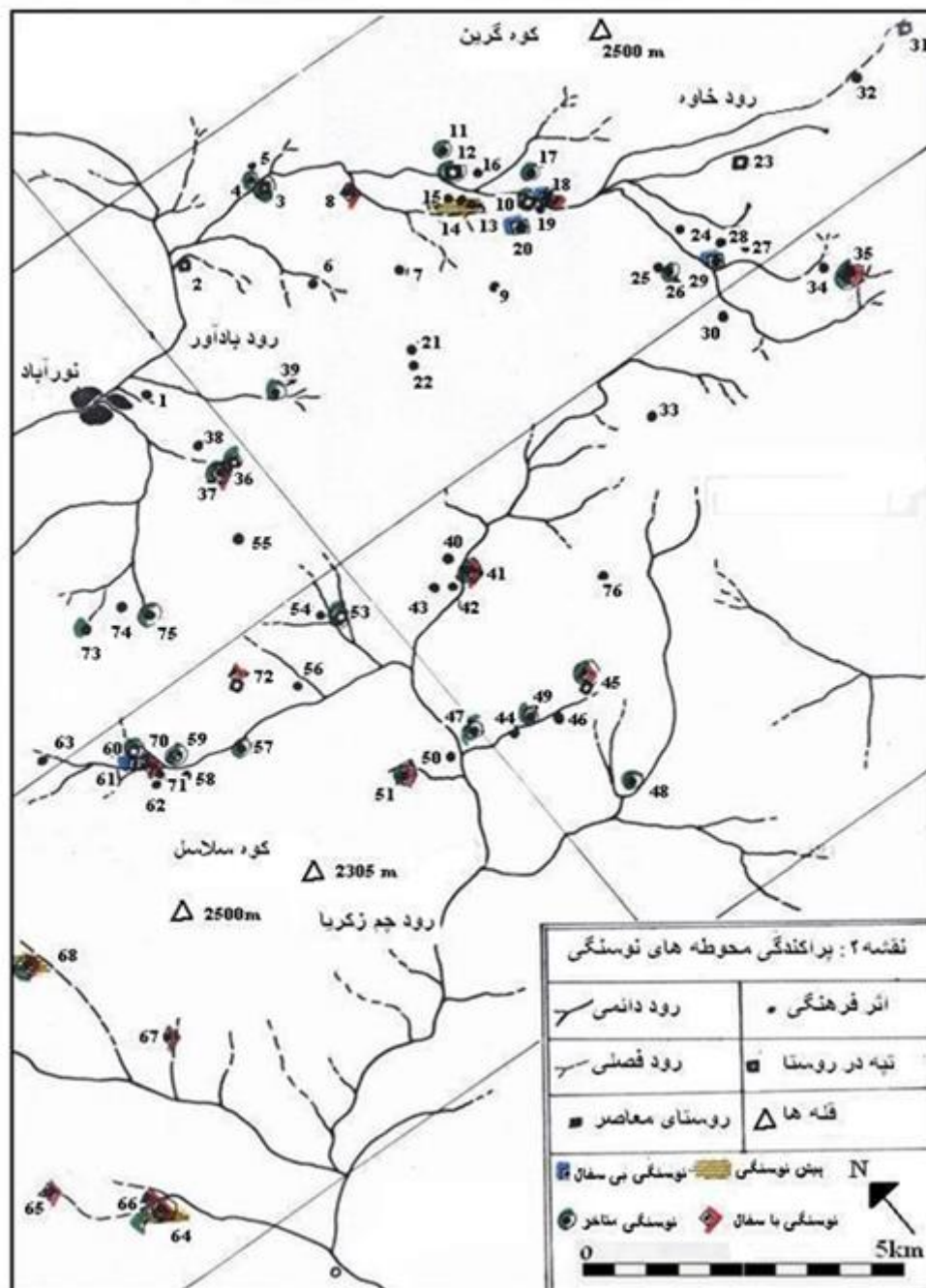
نقشه ۲: پراکندگی محوطه‌های نوسنگی
