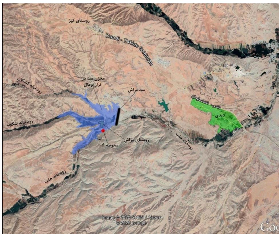
شکل ۳: جانمایی عمومی سد مخزنی مراش و حوضه آبرگیر آن (برگرفته از گوگل ارث)
