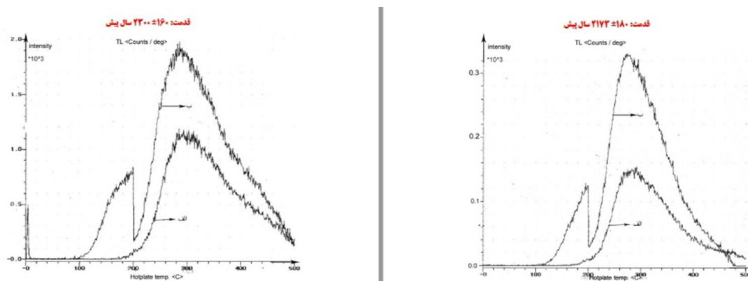
شکل ۹: نتایج ترمولومینسانس نمونه‌های مراش
