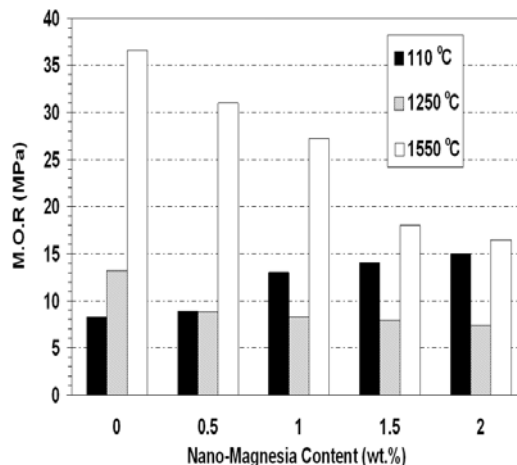
شکل ۵: تأثیر مقدار نانوذرات منیزیا بر استحکام خمشی سرد دیرگداز ریختنی کم سیمان پس از پخت در دماهای مختلف.
