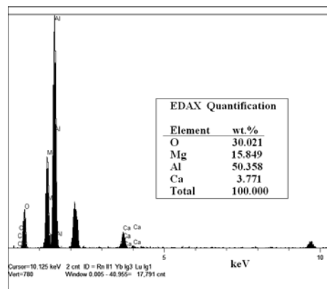
شکل ۱۱: آنالیز EDX ذرات اسپینل در ریزساختار دیرگداز ریختنی پخته شده در 1250^{\circ}\text{C} حاوی ۲ درصد وزنی نانوذرات منیزیا.
