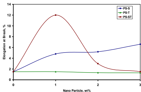
شکل ۵: تغییرات ازدیاد طول تا شکست نمونه‌های نانوکامپوزیتی با تغییر درصد نانوذرات.
