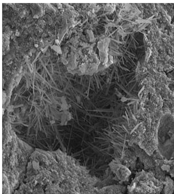
شکل (۲): جوانه زنی فاز سوزنی درون تخلخل در زمینه سیمانی
