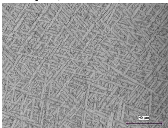
شکل (۷): ریز ساختار نمونه تغییر شکل یافته تا حد کرنش ۰/۵۵ در دمای ثابت 1000^{\circ}\text{C} و آهنگ کرنش 1 \times 10^{-2} \text{ s}^{-1} ، پس از باز پخت در دمای 980^{\circ}\text{C} به مدت ۲ ساعت در اتمسفر گاز خنثی.
