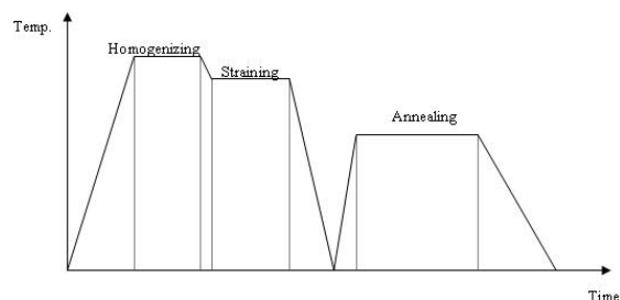
شکل (۱): سیکل شمتیک فرآیند اعمال شده روی آلیاژ Ti-6Al-4V در این تحقیق.
