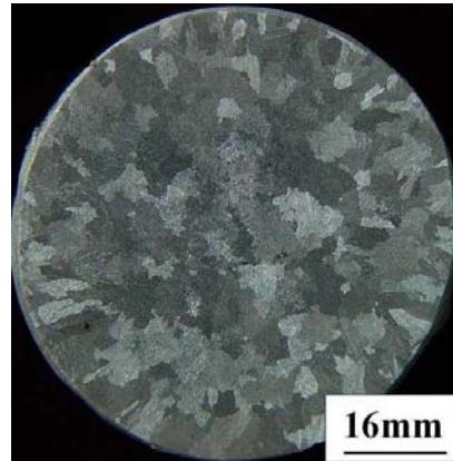
شکل (۳): تصویر ساختار میکروسکوپی نمونه ۱
