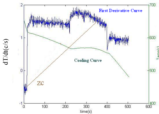
شکل (۴): منحنی سرد شدن به همراه مشتق اول آن و
