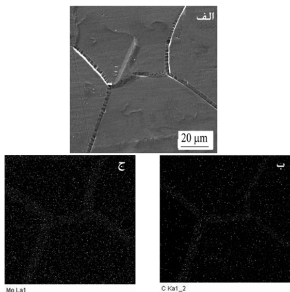
شکل (۸): الف- تصویر میکروسکپ الکترونی روبشی از فولاد حاوی 1/3 درصد مولیبدن، ب و ج: آنالیز سطحی کربن و مولیبدن در زمینه.
