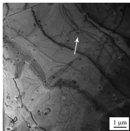
شکل (۷): کاربید \text{Mo}_2\text{C} تشکیل شده در نمونه حاوی 0/3 درصد مولیبدن.
