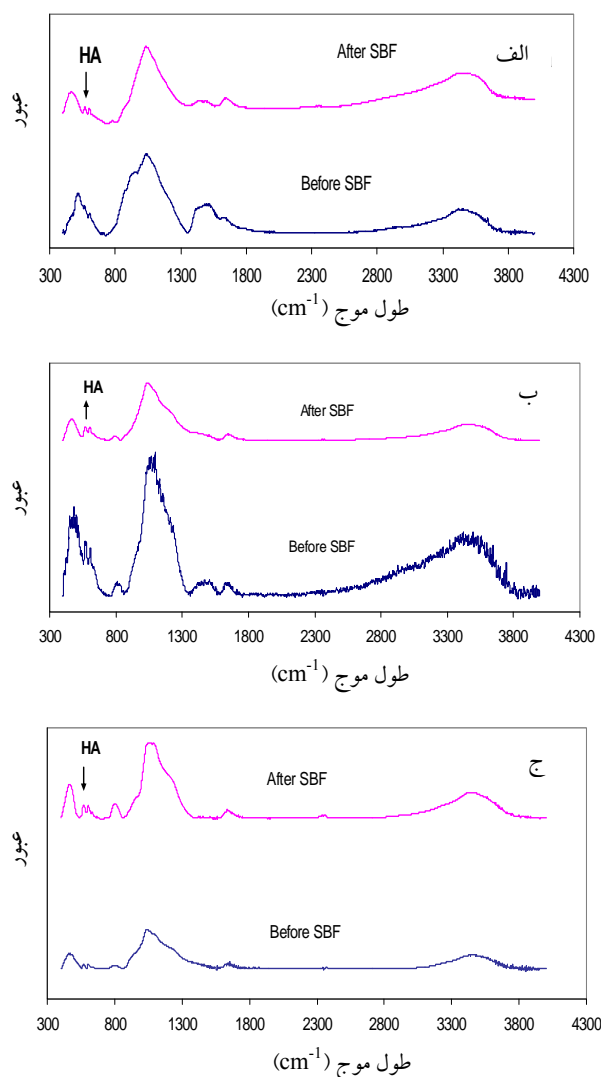
شکل (۶): طیف FTIR شیشه‌های زیست فعال، الف) ۴۵ S، ب) ۴۹ S و ج) ۵۸ S بعد از ۳۰ روز غوطه‌وری در محلول SBF.
