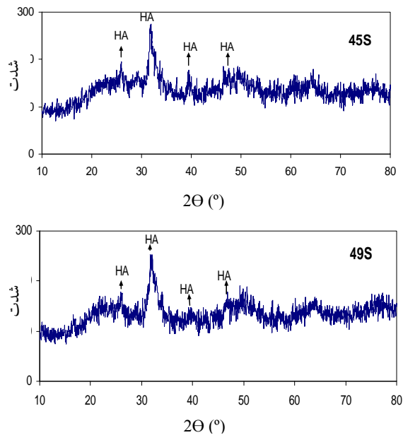
شکل (۳): الگوهای XRD پوشش‌های شیشه زیست فعال ۴۵ S و ۴۹ S بعد از ۳۰ روز غوطه‌وری در محلول SBF.
