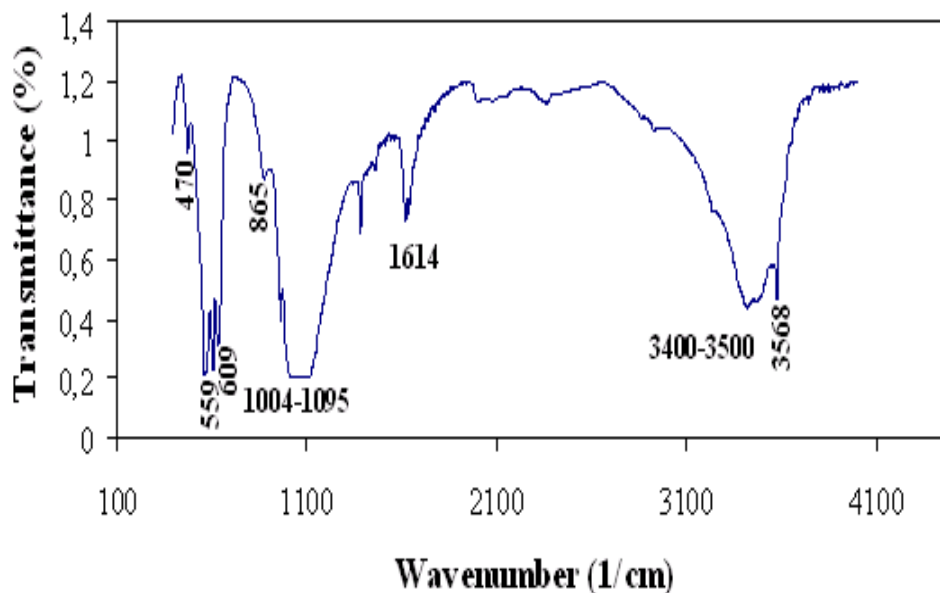
شکل (۶): طیف FTIR نمونه هیدروکسی آپاتیت سنتز شده با pH = 9.7 و دمای 150^\circ C و زمان ۲۴ ساعت.
