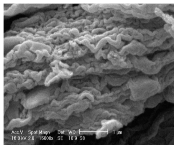
شکل (۱۷): تصویر تهیه شده توسط SEM از نانو ساختار \text{TiO}_2 بدست آمده از حرارت‌دهی الیاف چتایی ( 450^\circ\text{C} ) حاوی نانوذرات \text{TiO}_2 .
