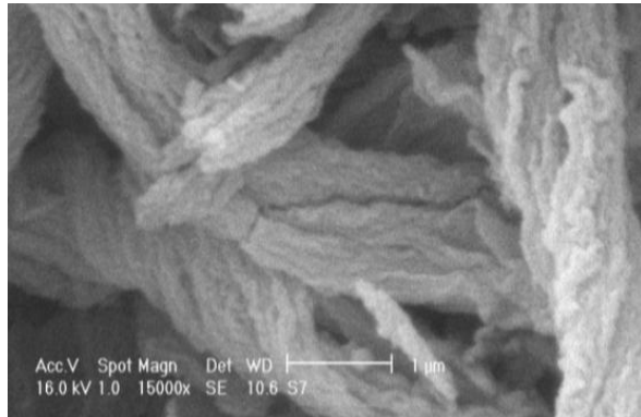
شکل (۱۴): تصویر تهیه شده توسط SEM از نانو فیبر \text{TiO}_2 بدست آمده از حرارت‌دهی الیاف پنبه ( 450^\circ\text{C} ) حاوی نانوذرات \text{TiO}_2 .
