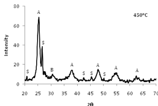
شکل (۳): منحنی XRD نمونه چتایی لایه‌نشانی شده با نانوذرات \text{TiO}_2 بدست آمده از محلول کلونیدی با \text{pH}=1/85 ، بعد از حرارت‌دهی در 450^\circ\text{C} . (A: Anatase, B: Brookite, R: Rutile, S: \text{SiO}_2 )
