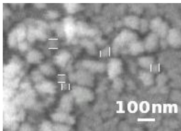
شکل ۵- تصویر تهیه شده توسط SEM پودر \text{TiO}_2 بدست آمده از محلول با \text{pH}=1/5 .
