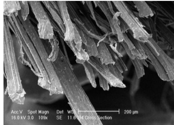
شکل (۱۲): تصویر تهیه شده توسط SEM از مقطع عرضی الیاف چتایی لایه‌نشانی شده (به مدت ۲۴ ساعت و دمای محیط) با نانوذرات \text{TiO}_2 موجود در محلول کلونیدی با \text{pH}=1/85 .
