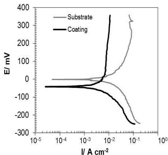
شکل (۳): نمودارهای پلاریزاسیون Tafel آلیاژ اینکونل 713C و پوشش آلومینایدی در نمک مذاب ( 70\text{Na}_2\text{SO}_4\text{-}25\text{NaCl}\text{-}5\text{V}_2\text{O}_5 (wt%) در دمای ۷۵۰ درجه سانتیگراد
