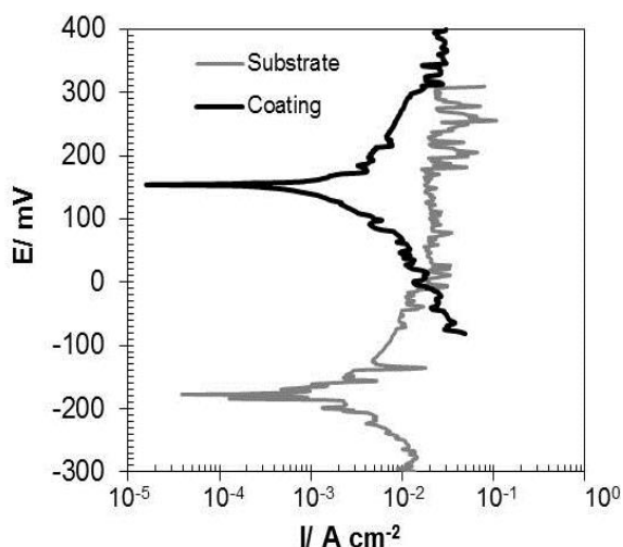
شکل (۴): نمودارهای پلاریزاسیون Tafel آلیاژ اینکونل 713C و پوشش آلومینایدی در نمک مذاب ( 70\text{Na}_2\text{SO}_4\text{-}30\text{NaCl} (wt%) در دمای ۷۵۰ درجه سانتیگراد
