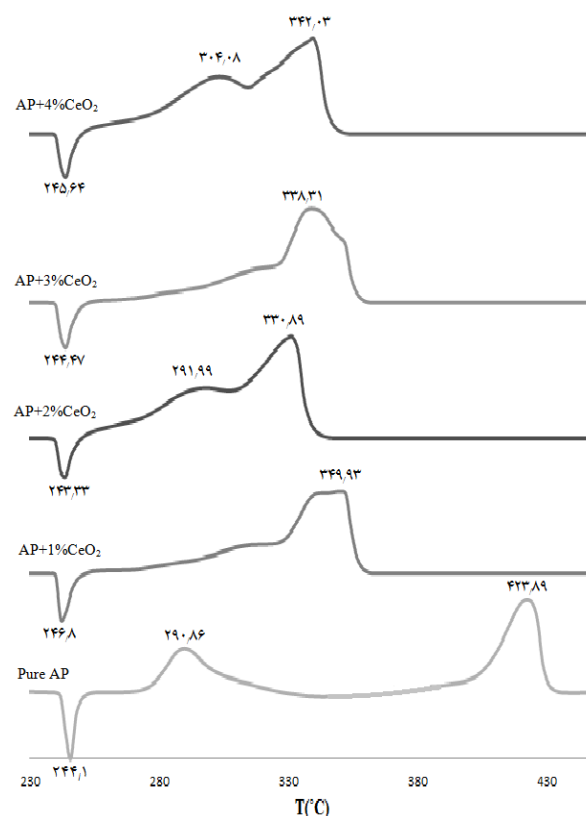
شکل (۴): منحنی‌های تجزیه گرمایی DSC (با سرعت گرمادهی 10^{\circ}C/min در اتمسفر هوا)
