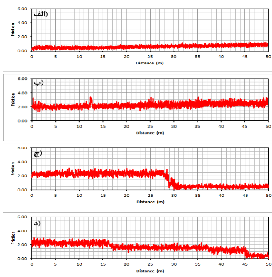
شکل (۳): اصطکاک بدست آمده از آزمون سایش برای پوشش های: (الف): تک لایه \text{TiO}_2 ، (ب): تک لایه HA، (ج): دو لایه HA- \text{TiO}_2 ، و (د): با ساختار تغییرات تدریجی HA/ \text{TiO}_2
