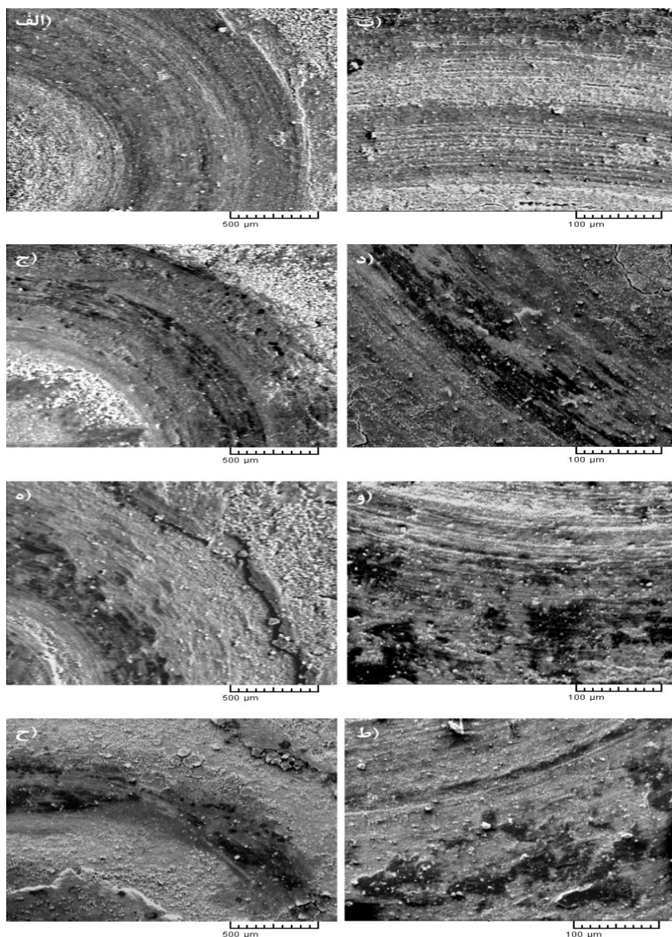
شکل (۲): تصاویر میکروسکوپ الکترونی از سطح سایش پوشش های: (الف و ب): تک لایه TiO_2 ، (ج و د): تک لایه HA، (ه و و): دو لایه HA- TiO_2 ، و (ح و ط): با ساختار تغییرات تدریجی HA/ TiO_2
