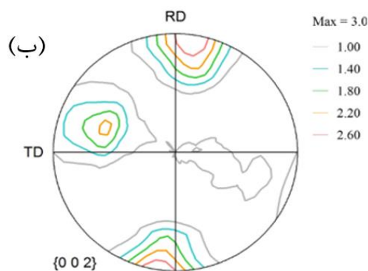
شکل (۵): تصویر قطبی نمونه اکستروژده شده شکل (۶): تصاویر قطبی نمونه های ED حاصل از آزمون فشار گرم در نرخ کرنش 1 s^{-1} و کرنش های: (الف): 0.06 و (ب): 0.1
