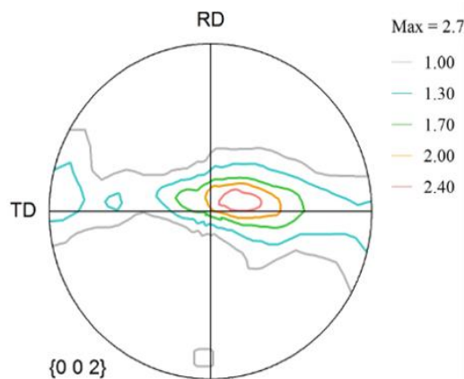
شکل (۵): تصویر قطبی نمونه اکستروژده شده
