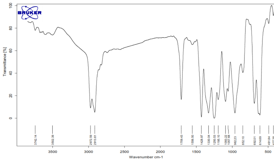
شکل (۳): طیف FT-IR پلی وینیل کلراید خالص
