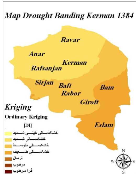
الف) کریجینگ
