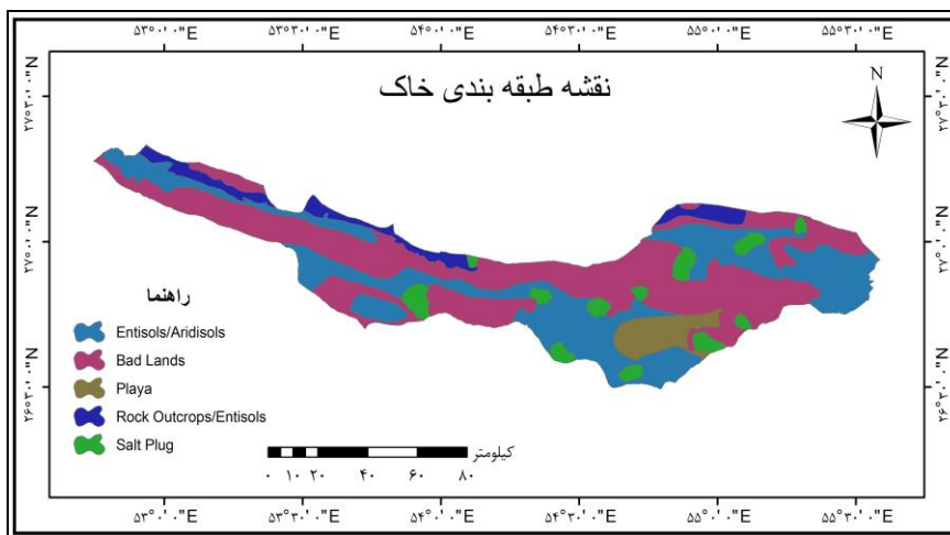
شکل ۵- نقشه طبقه بندی خاک شهرستان بندر لنگه - (منبع: نویسندگان، ۱۳۹۵)
