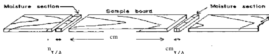
شکل ۱- روش بریدن نمونه کنترل و آزمونه‌های تعیین رطوبت
