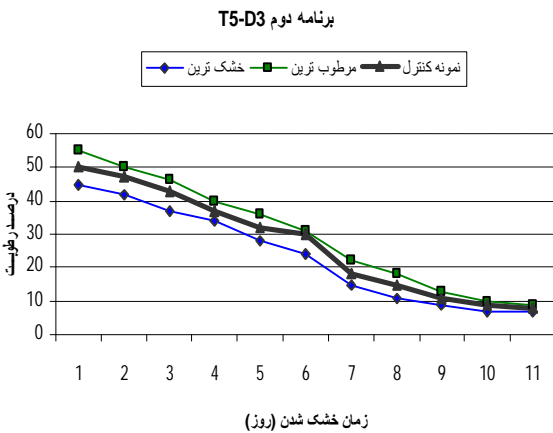
شکل 7- تغییرات رطوبت جاری بر حسب زمان در برنامه دوم
