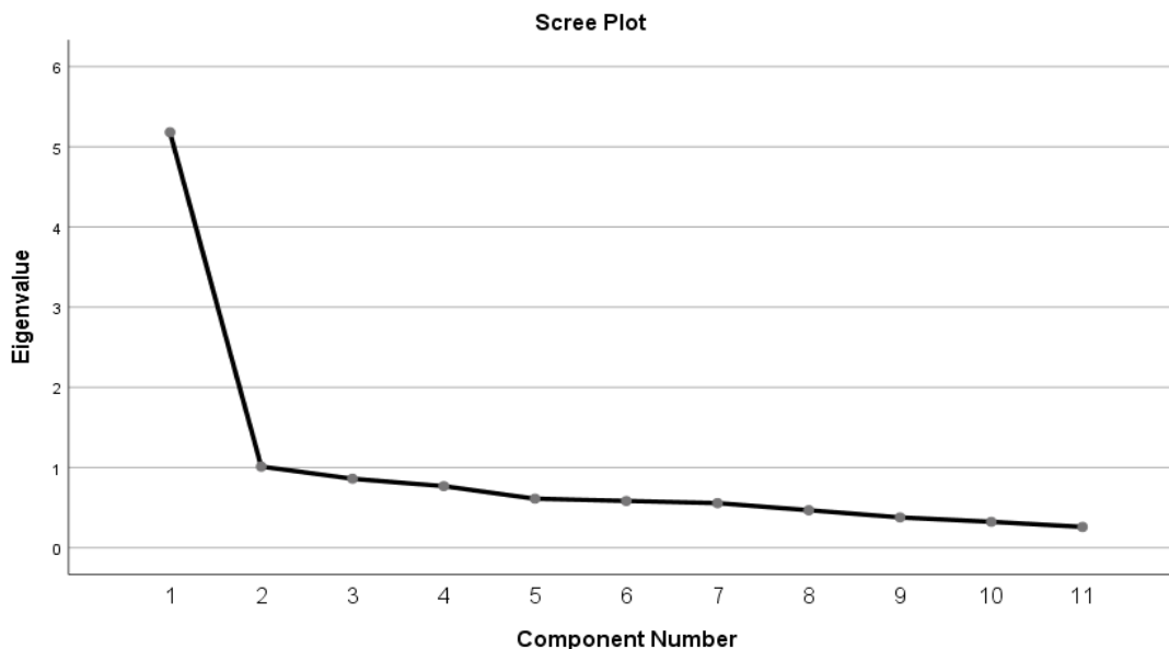
شکل ۱. نمودار اسکری کتل مولفه‌های استخراجی مقیاس هیجان‌خواهی جنسی
