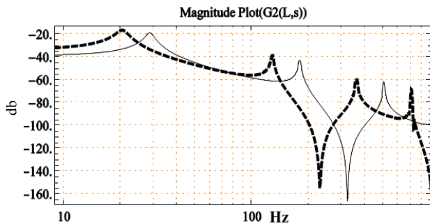
شکل (۵): پاسخ فرکانسی برای تابع تبدیل مربوط به نیروی هارمونیک گسترده برای مقادیر مختلف عرض تیر (b → 0.005 , dashed line), (b → 0.01 , solid line) و سایر ورودی های h \rightarrow 0.2 * 10^{-3}, L \rightarrow 0.04, \tau \rightarrow 10^6, C \rightarrow 0.5
