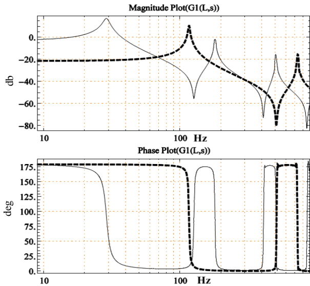
شکل (۶): نمودارهای بود مربوط به تابع تبدیل در صورت اعمال نیروی متمرکز هارمونیک در سر آزاد تیر را برای مقادیر مختلف (L → 0.02 , dashed line), (L → 0.04 , solid line) و سایر ورودی های b \rightarrow 0.01, h \rightarrow 0.2 * 10^{-3}, \tau \rightarrow 10^6, C \rightarrow 0.5
