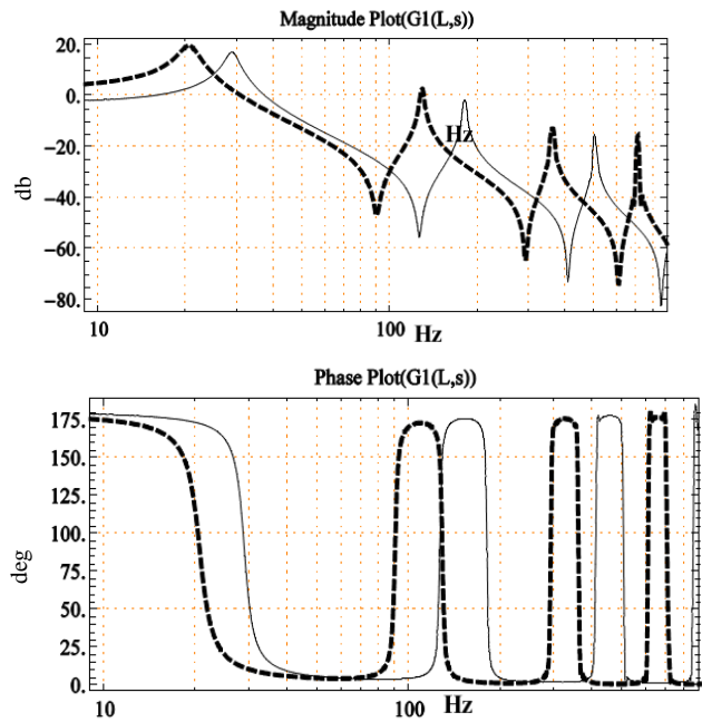
شکل (۴): نمودارهای بود مربوط به تابع تبدیل در صورت اعمال نیروی متمرکز هارمونیک در سر آزاد تیر را برای مقادیر مختلف عرض تیر (b → 0.005 , dashed line), (b → 0.01 , solid line) و ورودی C \rightarrow 0.5
