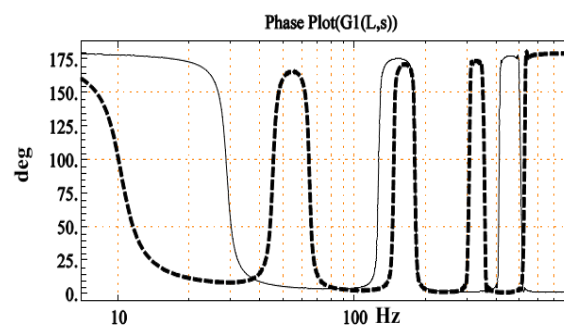
شکل (۸): نمودارهای بود مربوط به تابع تبدیل در صورت اعمال نیروی متمرکز هارمونیک در سر آزاد تیر برای مقادیر مختلف ارتفاع تیر (h \rightarrow 0.1 * 10^{-3}, \text{dashed line}) , (h \rightarrow 0.2 * 10^{-3}, \text{solid line}) اندازه پاسخ فرکانسی را برای تابع تبدیل مربوط به نیروی هارمونیک گسترده را برای مقادیر مختلف ارتفاع تیر را در شکل (۹) داریم:
