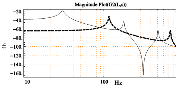
شکل (۷): پاسخ فرکانسی را برای تابع تبدیل مربوط به نیروی هارمونیک گسترده را برای مقادیر مختلف طول تیر (L → 0.02 , dashed line), (L → 0.04 , solid line) و سایر ورودی های b \rightarrow 0.01, h \rightarrow 0.2 * 10^{-3}, \tau \rightarrow 10^6, C \rightarrow 0.5
