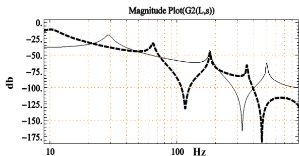
شکل (۹): پاسخ فرکانسی برای تابع تبدیل مربوط به نیروی هارمونیک گسترده
