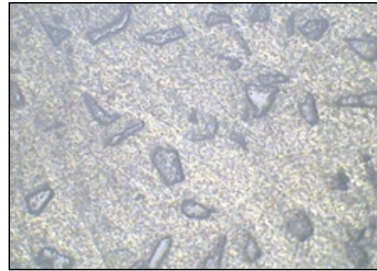
شکل (۳) نحوه توزیع ذرات کاربید سیلیسیم در داخل کامپوزیت.
