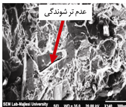
شکل (۶) عدم ترشوندگی مناسب ذرات توسط آلومینیم در سطح شکست.
