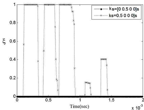
شکل (۱۱) تأثیر موقعیت قرارگیری سیم‌های حافظه‌دار در تغییرات کسر حجمی مارتنزیت
