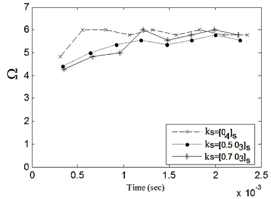
شکل (۹) تغییرات فرکانس طبیعی \Omega = \omega a^2 (\rho/h^2 E_2)^{1/2} برای کسر حجمی‌های متفاوت
