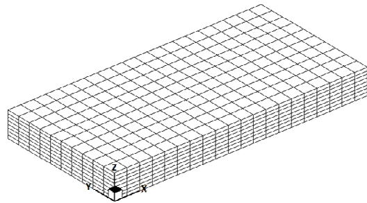
شکل (۱۷) شبکه غیر منطبق بر مرز مورد استفاده در حل مسئله ورق سوراخدار
