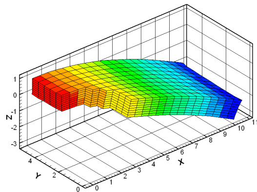
شکل (۱۸) نمای تغییر شکل یافته ورق سوراخدار با استفاده از روش بهبود یافته المان محدود شبکه ثابت
