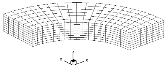
شکل (۷) شبکه منطبق بر مرز برای تحلیل تیر خمیده به روش المان محدود استاندارد
