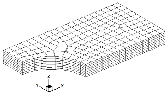
شکل (۱۵) شبکه منطبق بر مرز مورد استفاده در تحلیل المان محدود ورق سوراخدار
