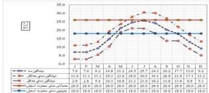
شکل ۵. نمودار حدود منطقه آسایش در شهر رشت
