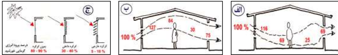
شکل ۸. نقش انواع سایه‌سازها در کاهش انرژی گرمایی خورشید و بهبود وضعیت دمای داخل فضاهای مسکونی (ا.ج. اوتز، ۱۳۷۴)
