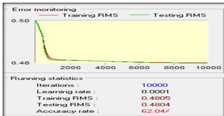
شکل ۱۱. ارزیابی صحت شبکه عصبی مصنوعی پرسپترون (MLP)
