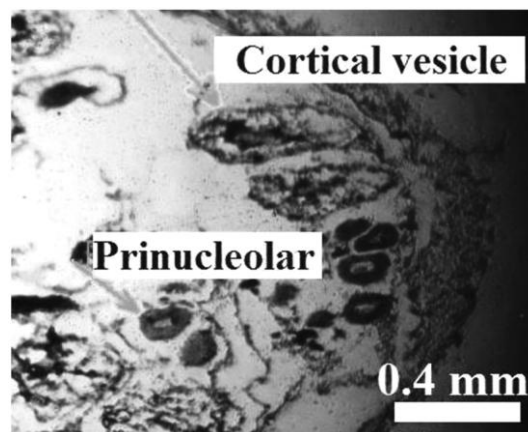
شکل ۲- مرحله ۳، زرده‌سازی اولیه، تخمک‌هایی با رشد اولیه و کورتیکال آلفونولی مشاهده شد.
