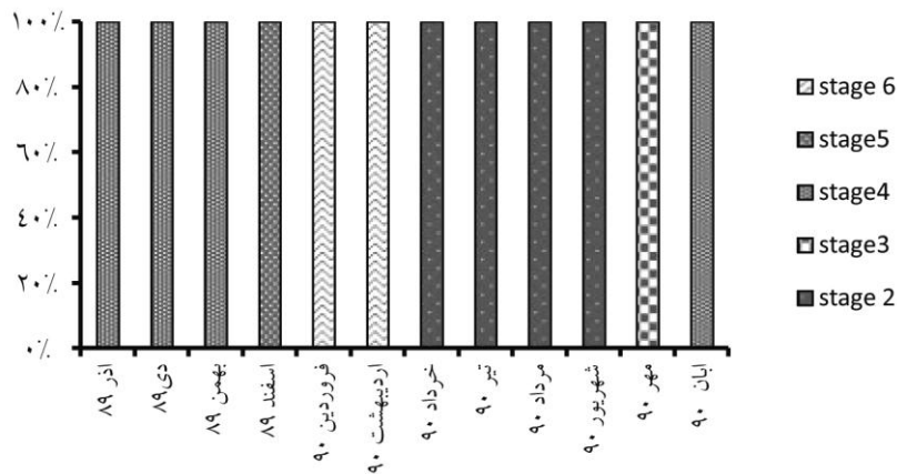
شکل ۶- فراوانی مراحل رسیدگی جنسی گنادهای ماهی سوف حاجی‌طرخان تالاب امیرکلاهی.
