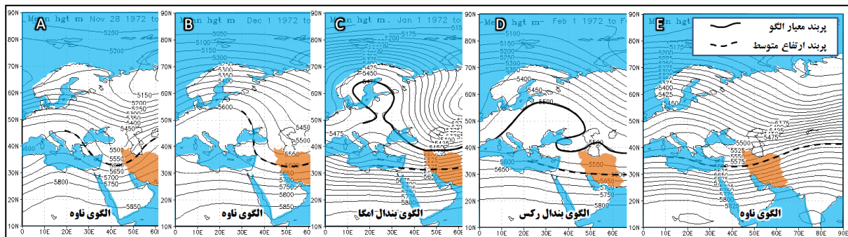
شکل ۶: الگوی همید سامانه مؤثر بر طولانی‌ترین دوره دماهای صفر و زیر صفر ایران و رخداد رکوردهای سرما از ۲۸ نوامبر تا ۲۹ مارس ۱۹۷۲
