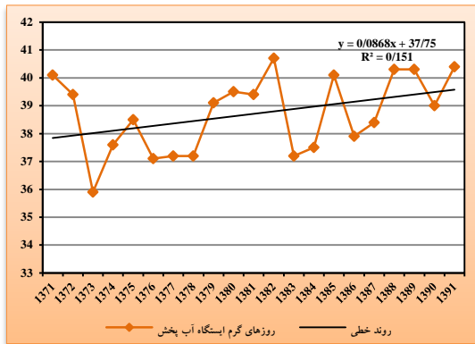
شکل ۲۳: نمودار روند خطی نمایه روزهای گرم ایستگاه آب پخش طی دوره آماری ۱۳۷۱-۱۳۹۱
