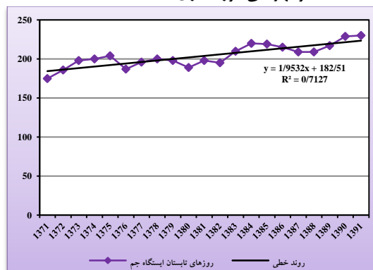
شکل ۴۲: نمودار روند خطی نمایه روزهای تابستان ایستگاه جم طی دوره آماری ۱۳۷۱-۱۳۹۱
