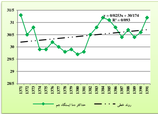
شکل ۷: نمودار روند خطی تغییرات میانگین حداکثر دمای سالانه ایستگاه جم طی دوره آماری ۱۳۷۱-۱۳۹۱
