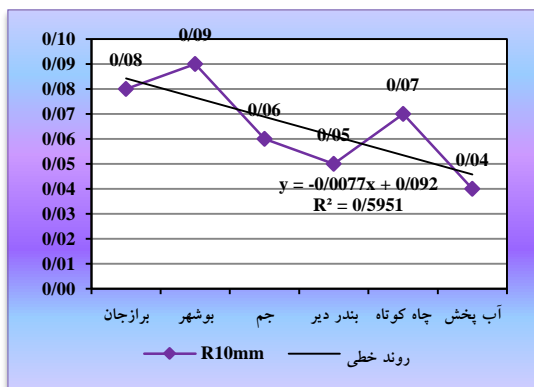
شکل ۵۳: نمودار روند خطی تعداد روزهایی با بارش سنگین ایستگاه‌های مورد مطالعه طی دوره آماری ۱۳۷۱-۱۳۹۱
