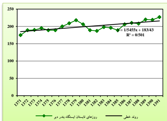
شکل ۳۹: نمودار روند خطی نمایه روزهای تابستان ایستگاه بندر دیر طی دوره آماری ۱۳۷۱-۱۳۹۱
