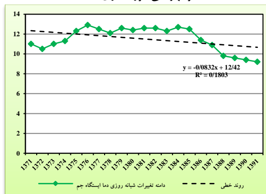
شکل ۴۸: نمودار روند خطی نمایه دامنه تغییرات شبانه روزی دما ایستگاه جم طی دوره آماری ۱۳۷۱-۱۳۹۱
