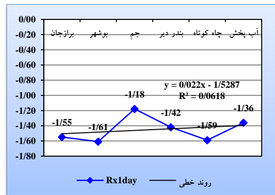
شکل ۵۰: نمودار روند خطی حداکثر بارش یک روزه ایستگاه‌های مورد مطالعه طی دوره آماری ۱۳۷۱-۱۳۹۱
