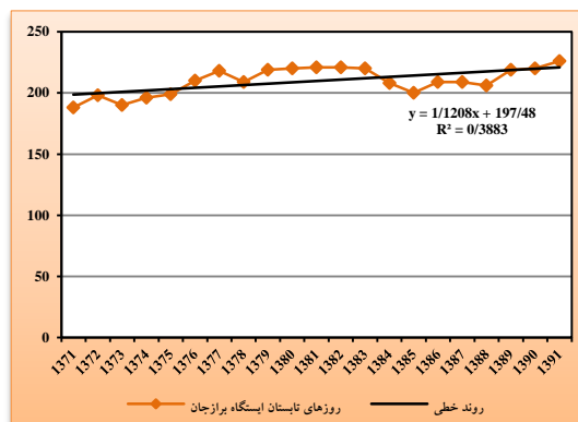
شکل ۳۸: نمودار روند خطی نمایه روزهای تابستان ایستگاه برازجان طی دوره آماری ۱۳۷۱-۱۳۹۱
