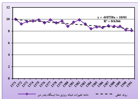
شکل ۴۵: نمودار روند خطی نمایه دامنه تغییرات شبانه روزی دما ایستگاه بندر دیر طی دوره آماری ۱۳۷۱-۱۳۹۱
