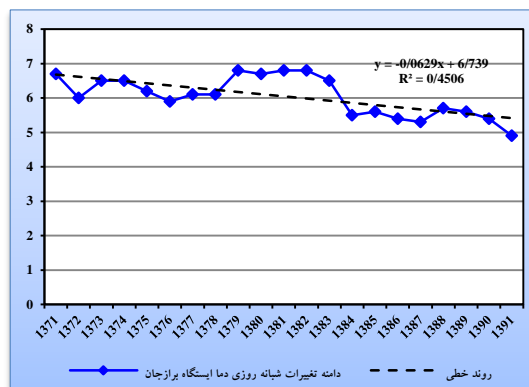
شکل ۴۴: نمودار روند خطی نمایه دامنه تغییرات شبانه روزی دما ایستگاه برازجان طی دوره آماری ۱۳۷۱-۱۳۹۱
