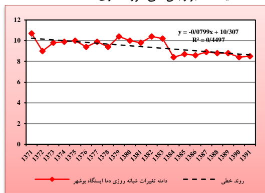
شکل ۴۶: نمودار روند خطی نمایه دامنه تغییرات شبانه روزی دما ایستگاه بوشهر طی دوره آماری ۱۳۷۱-۱۳۹۱
