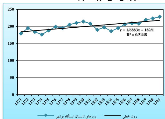
شکل ۴۰: نمودار روند خطی نمایه روزهای تابستان ایستگاه بوشهر طی دوره آماری ۱۳۷۱-۱۳۹۱
