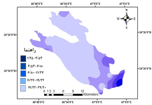
شکل ۵: نقشه سطح پیژومتری منطقه قبل از احداث کانال، سال ۱۳۸۷
