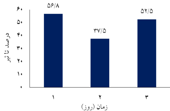
نمودار ۳: تاثیر سطوح مختلف زمان بر فروشوی طلای مقاوم.
