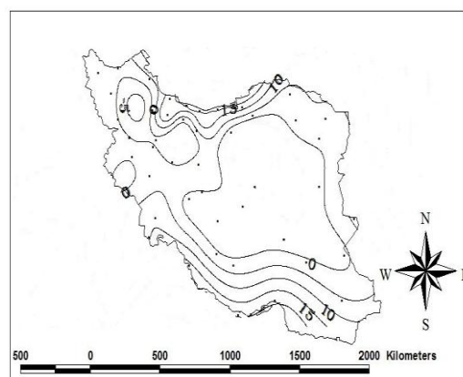
شکل ۱۴- میانگین دمای نقطه شبنم سالانه (درجه سانتی گراد در سه سال) طی دوره آماری ۱۹۷۶-۲۰۰۵
