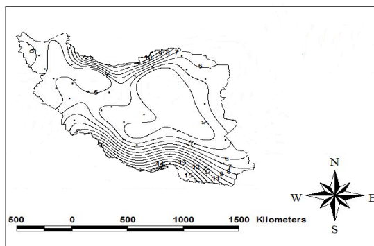
شکل ۳- میانگین رطوبت ویژه سالانه (گرم بر
