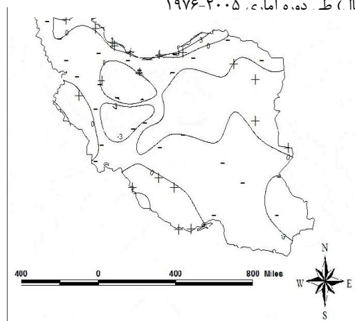
شکل ۱۲- روند رطوبت ویژه فصل تابستان (JJA) (گرم بر کیلو گرم در سه سال) طی دوره آماری ۱۹۷۶-۲۰۰۵
