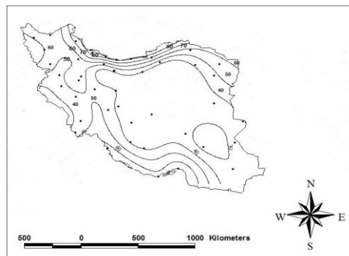
شکل ۲- میانگین رطوبت نسبی سالانه (درصد) طی
