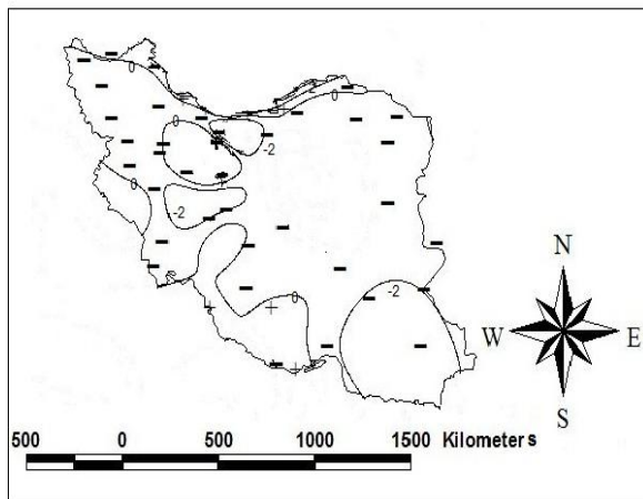
شکل ۱۱- روند رطوبت ویژه فصل بهار (MAM) (گرم بر کیلو گرم در سه سال) طی دوره آماری ۱۹۷۶-۲۰۰۵
