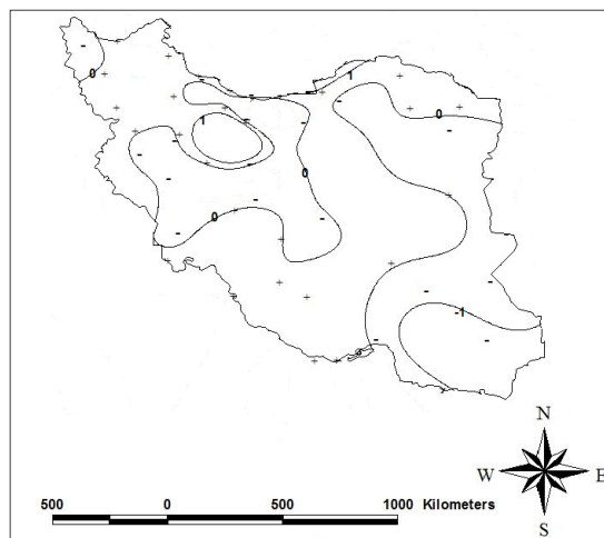
شکل ۱۰- روند رطوبت نسبی فصل زمستان (DJF) بر حسب (درصد درسی سال) طی دوره آماری ۱۹۷۶-۲۰۰۵
