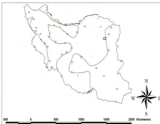
شکل ۱۵- روند دمای نقطه شبنم سالانه (درجه سانتی گراد در سه سال) طی دوره آماری ۱۹۷۶-۲۰۰۵
