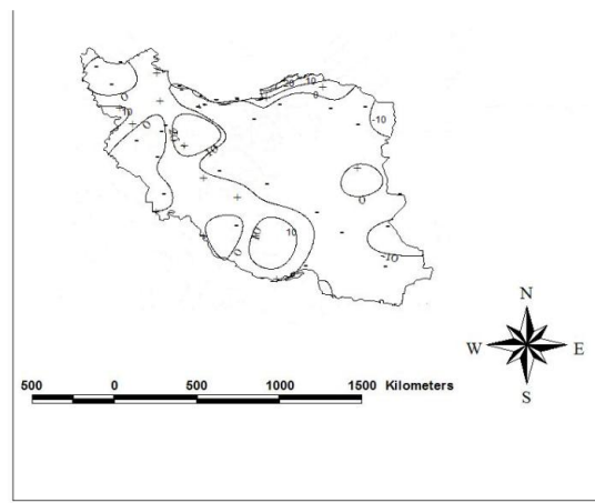
شکل ۶- روند رطوبت نسبی فصل زمستان (DJF) (درصد درسی سال) طی دوره آماری ۱۹۷۶-۲۰۰۵
