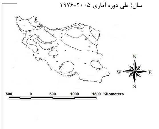
شکل ۹- روند رطوبت نسبی فصل پاییز (SON) (درصد در سی سال) طی دوره آماری ۱۹۷۶-۲۰۰۵
