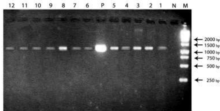
شکل ۳- نتیجه واکنش زنجیره ای پلی مرز روی ژل آگارز ۱/۵٪، M خط کش مولکولی ۱ کیلو بازی، P کنترل مثبت، ۱-۱۲ نمونه های آرکوباکتر جدا شده، N کنترل منفی
