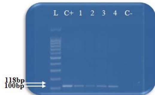
شکل ۲- شناسایی سویا در محصولات سوسیس (L: 1000-100 bp Ladder، C+: کنترل مثبت پرایمر سویا، ۱: سوسیس برند A، ۲: سوسیس برند B، ۳: سوسیس برند C، ۴: سوسیس برند D، C-: کنترل منفی)
