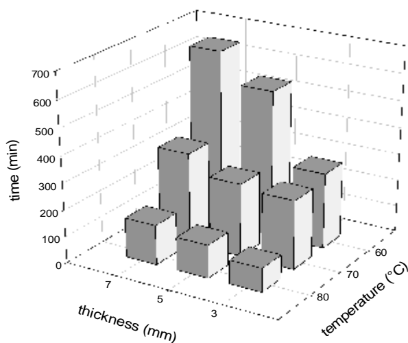
شکل 5- اثر ضخامت تیغه‌ها بر زمان خشک کردن در دمای 60، 70 و 80 درجه‌ی سانتی‌گراد
