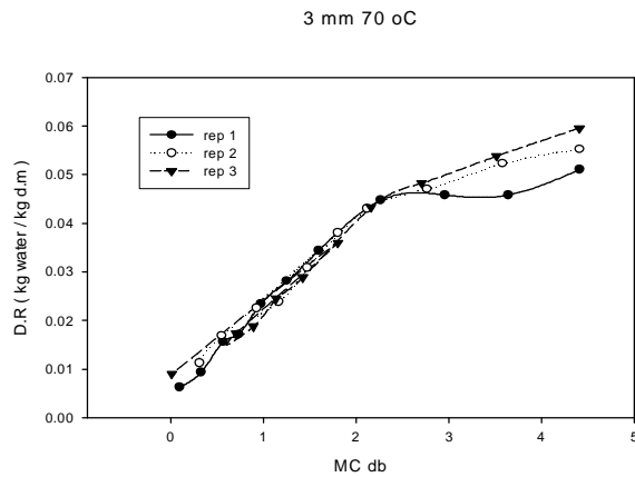
شکل 6- مقایسه‌ی نقطه‌ی شکست سه تکرار ضخامت 3 mm در دمای 70° C
