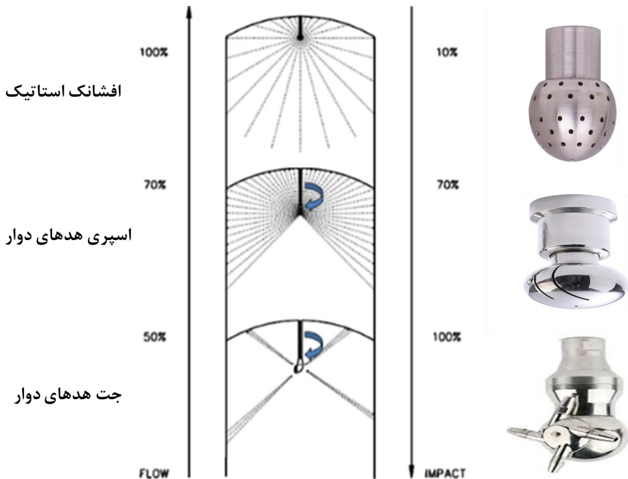
شکل (۴) - دبی، میزان برخورد و پوشش توسط انواع افشانک‌ها
