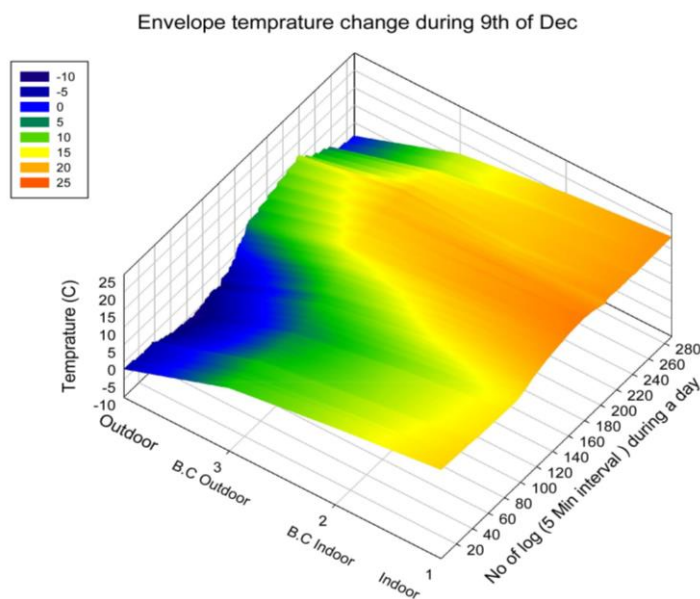
نمودار ۷- نمودار سه بعدی دمای لحظه ای سطوح مختلف در یک روز، ساختمان سعیدییه
