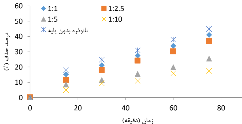
شکل ۴- مقایسه فعالیت سونوفتوکاتالیزوری نانوکامپوزیت‌ها با نسبت‌های مختلف
