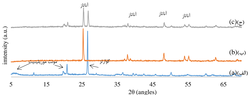
شکل ۳- الگوی XRD بنتونیت (الف)، نانوذرات دی‌اکسیدتیتانیوم (ب)، نانوکامپوزیت بنتونیت/دی‌اکسیدتیتانیوم تهیه شده با نسبت مقدار تیتانیا به بنتونیت ۱: ۲/۵ (ج).
