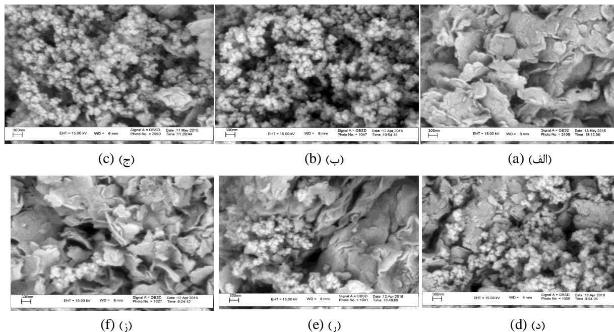
شکل ۱- تصاویر میکروسکوپ الکترونی بنتونیت (الف)، نانوذرات دی‌اکسیدتیتانیوم (ب)، نانوکامپوزیت بنتونیت/دی‌اکسیدتیتانیوم تهیه شده با نسبت مقدار تیتانیا به بنتونیت ۱:۱ (ج)، ۲/۵:۱ (د)، ۵:۱ (ر) و ۱۰:۱ (ز).
