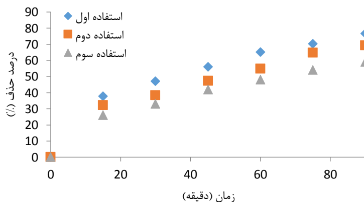
شکل ۸- بررسی امکان استفاده مجدد فتوکاتالیست بر راندمان حذف
