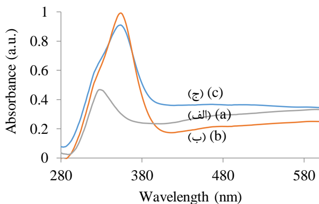
شکل ۲- طیف جذب نور بنتونیت (الف)، نانوذرات دی‌اکسیدتیتانیوم (ب)، نانوکامپوزیت بنتونیت/دی‌اکسیدتیتانیوم تهیه شده با نسبت مقدار تیتانیا به بنتونیت ۱: ۲/۵
