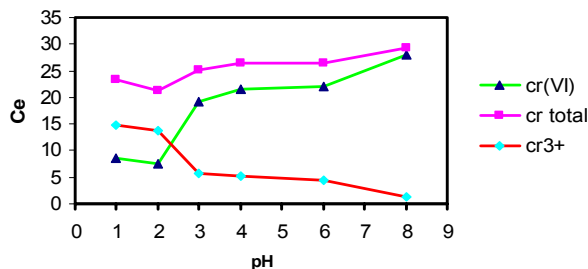
نمودار ۲- اثر تغییرات pH بر جذب Cr(VI) و کل کروم Cr(III)
